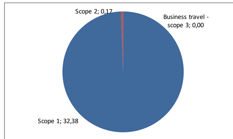
Scopes in cirkeldiagram
